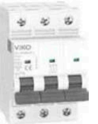
6 kA 3 Kutup Otomatik Sigorta C Tipi
